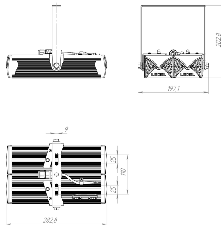
Рисунок 1 Габаритные размеры светильника «СВ-36»
