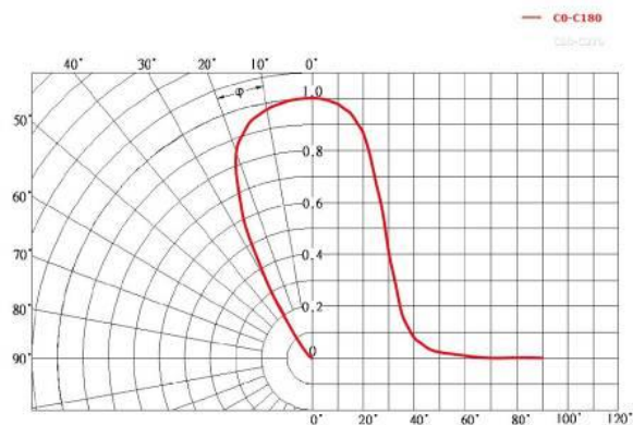
Рисунок 3 Тип КСС
